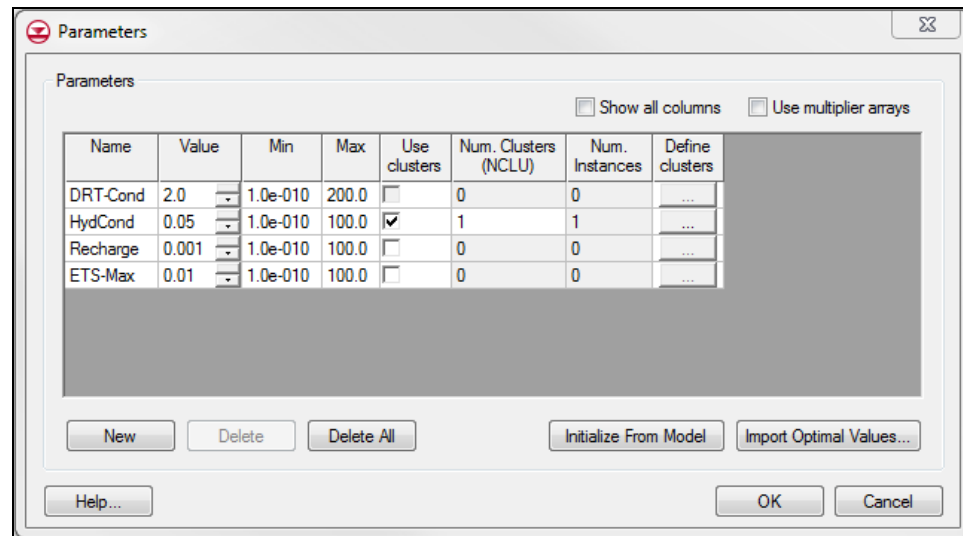
Figure 11 MODFLOW parameters
